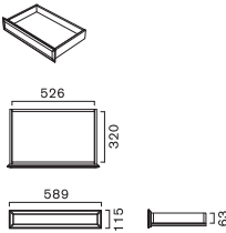
Mタイプ (W589)
