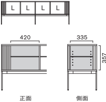
Lタイプ (W420)
