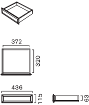
Sタイプ (W436)
