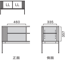
LLタイプ (W460)
