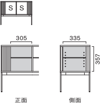
Sタイプ (W305)
