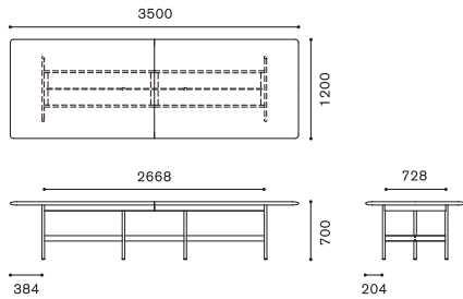
W3500×D1200×H700
