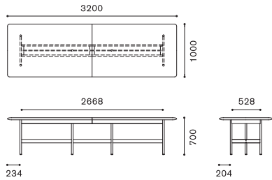
W3200×D1000×H700
