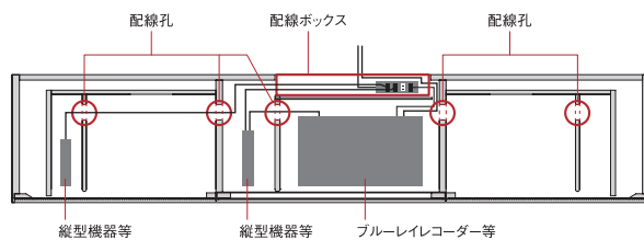
断面図(上面)
