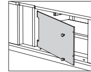
バックプレートの右端のネジを外し、プレートを右斜め手前側に引き、取り外します。
