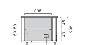
断面図 C-C
