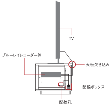
断面図(側面)
