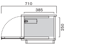
断面図 A-A
