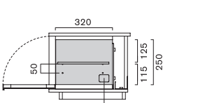
断面図 B-B
