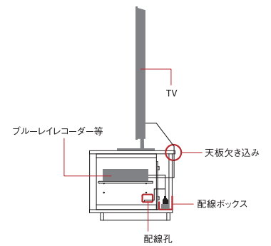
断面図(側面)
