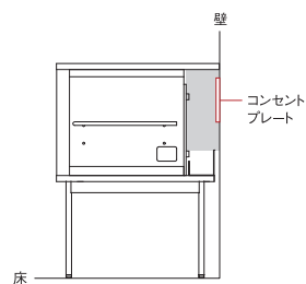
断面図(側面)
